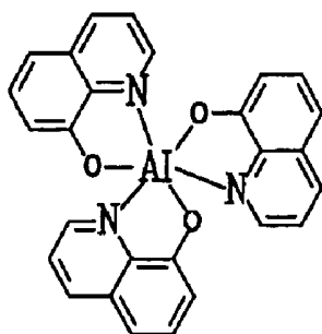
Alq 3
