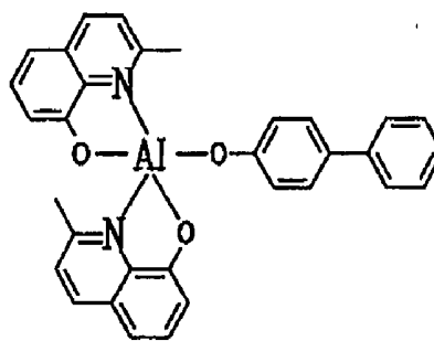
BAlq
